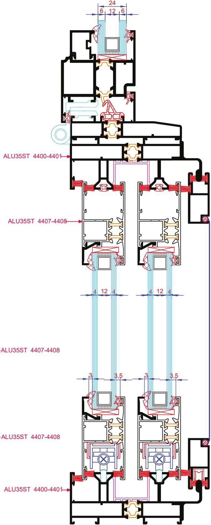
Üstü Kanat Detayı
